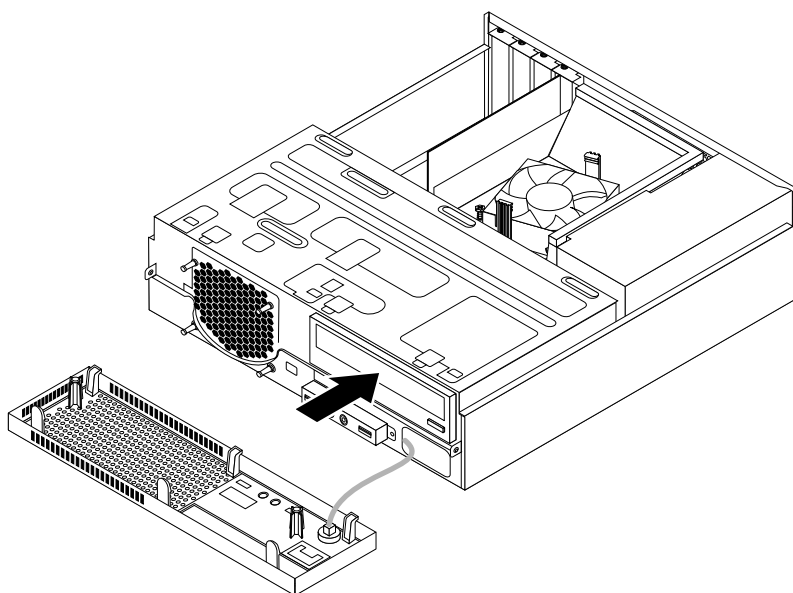
Obrázek 27. Instalace nové optické jednotky
