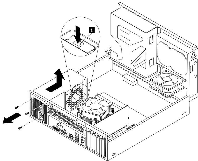
Obrázek 31. Odstranění napájecího zdroje
