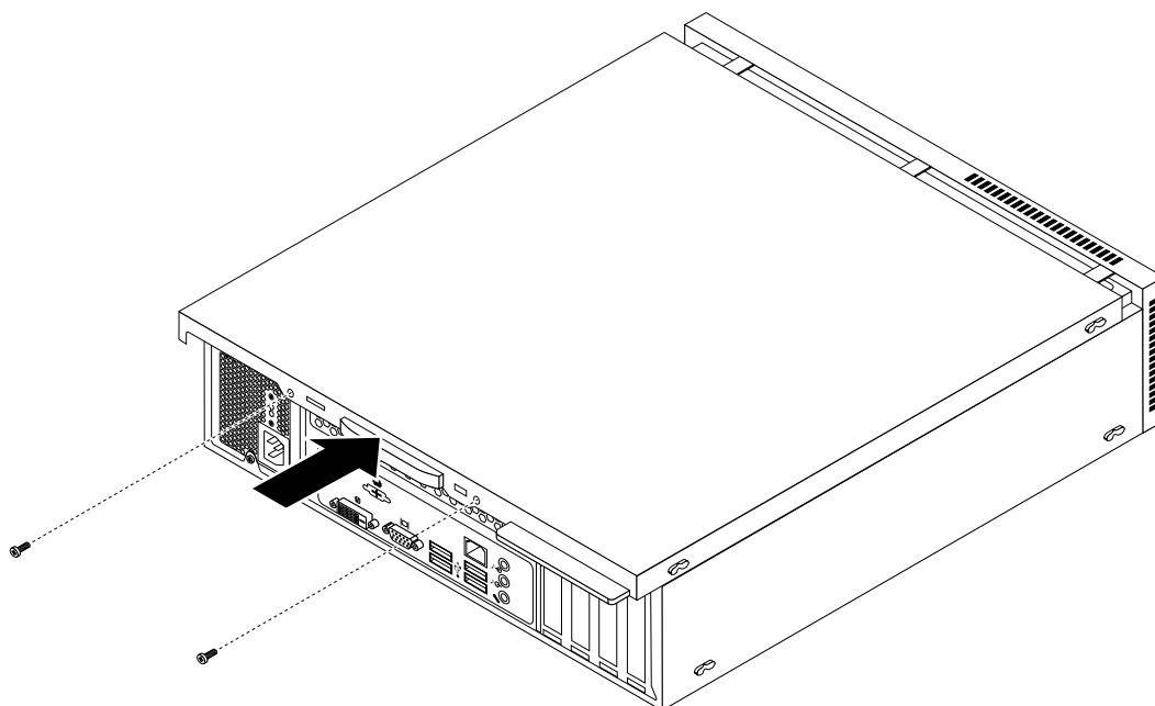
Obrázek 44. Instalace krytu počítače
