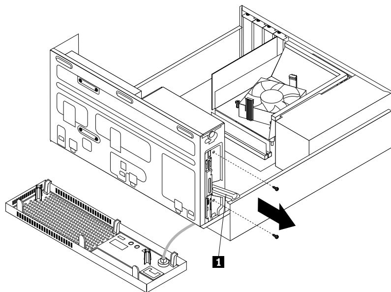
Obrázek 24. Odstranění optické jednotky
