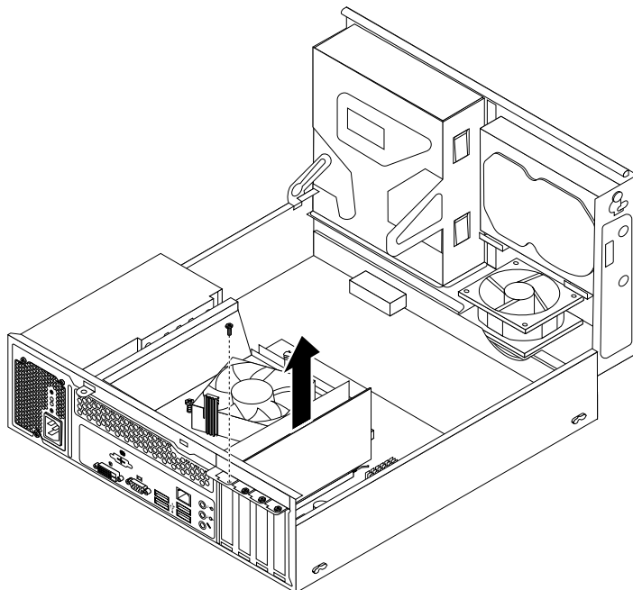
Obrázek 14. Odstranění karty PCI
