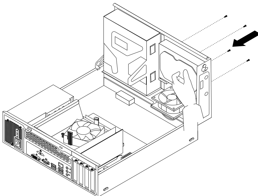
Obrázek 23. Instalace jednotky pevného disku
