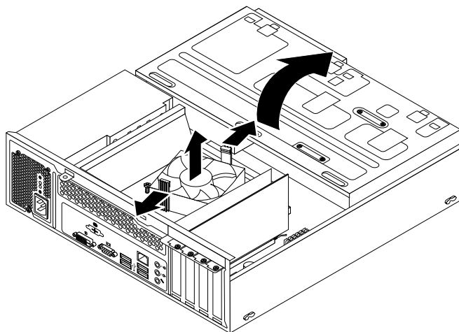
Obrázek 34. Vyjmutí vedení chladiče a větráku
