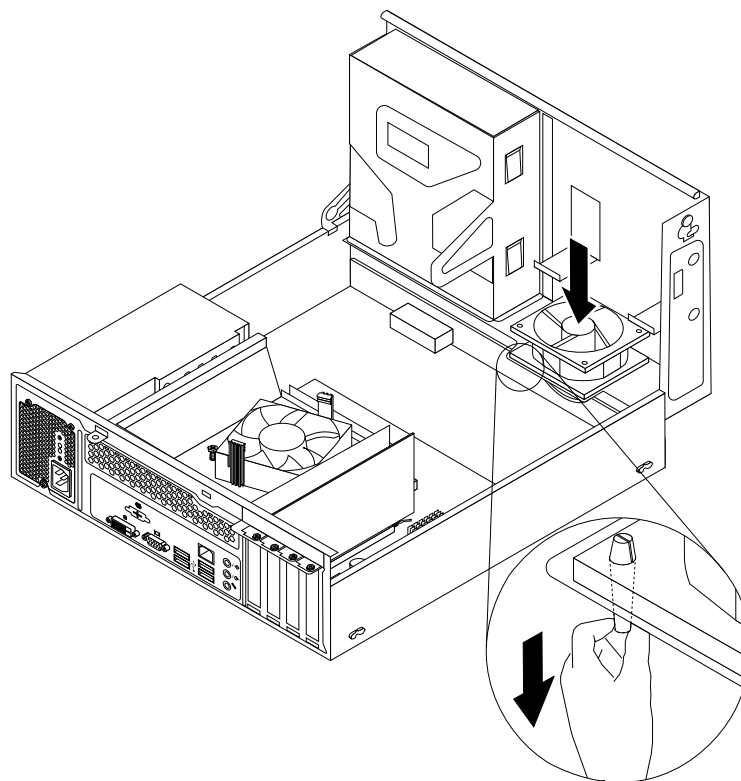
Obrázek 41. Instalace sestavy větráku systému
