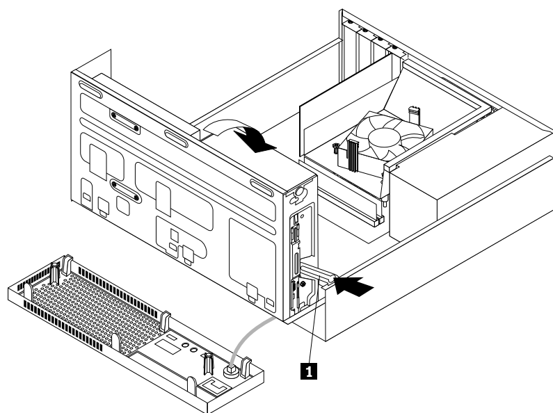
Obrázek 25. Sklopení sestavy pozice jednotky
