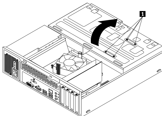
Obrázek 20. Odklopení sestavy pozic jednotek
