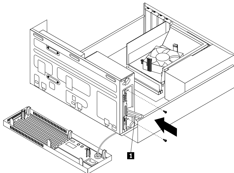
Obrázek 28. Instalace optické jednotky
