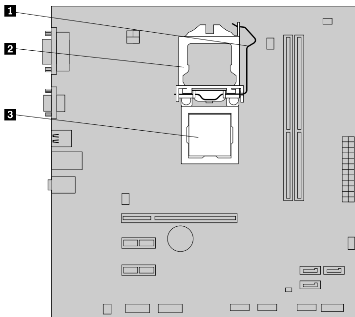
Obrázek 37. Přístup k mikroprocesoru
