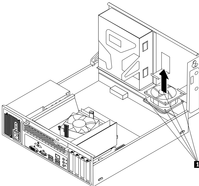
Obrázek 40. Odstranění sestavy větráku systému
