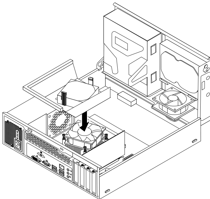
Obrázek 33. Instalace vedení chladiče a větráku
