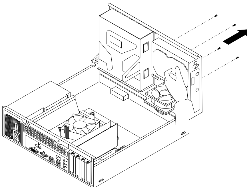
Obrázek 21. Odstranění jednotky pevného disku
