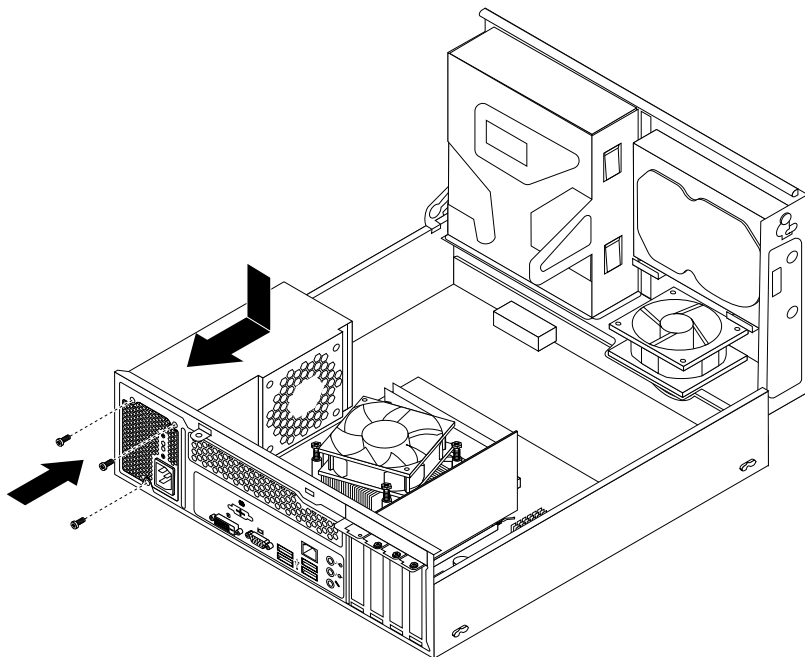
Obrázek 32. Instalace sestavy napájecího zdroje
