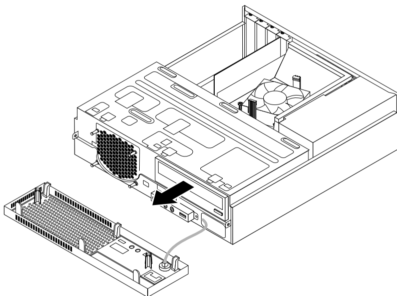
Obrázek 26. Odstranění optické jednotky
