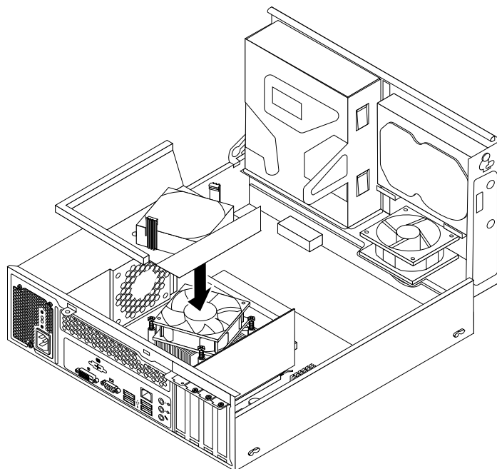
Obrázek 36. Instalace vedení chladiče a větráku
