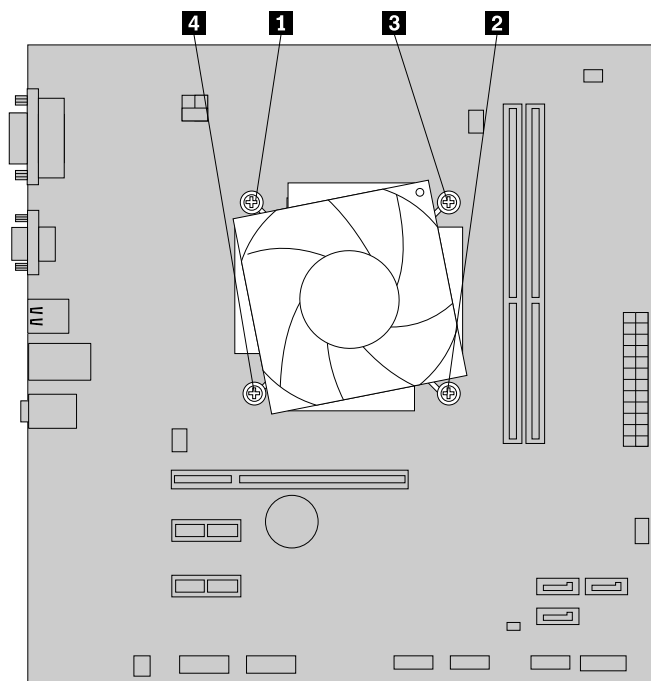
Obrázek 35. Odstranění sestavy chladiče a větráku
