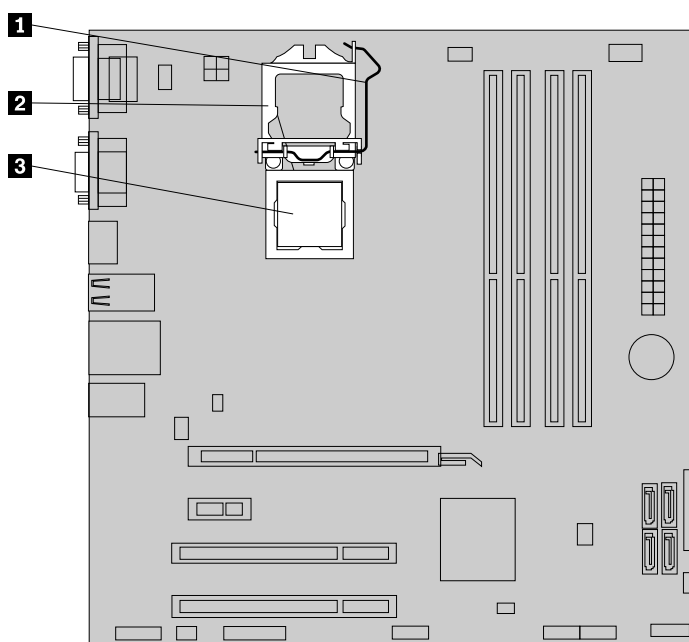
Obrázek 41. Přístup k mikroprocesoru
