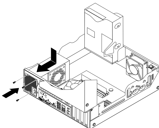
Obrázek 39. Instalace sestavy napájecího zdroje
