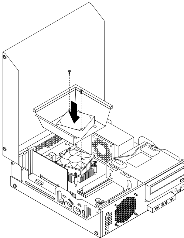
Obrázek 35. Instalace vedení chladiče a větráku
