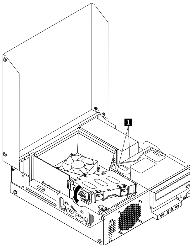
Obrázek 28. Instalace jednotky pevného disku
