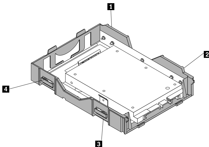
Obrázek 25. Instalace jednotky SSD s redukcí úložiště do rámečku jednotky pevného disku
