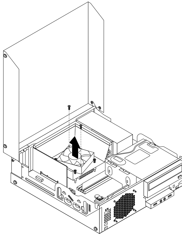
Obrázek 36. Vyjmutí vedení chladiče a větráku
