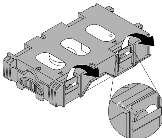
Obrázek 27. Vyjmutí jednotky pevného disku z rámečku
