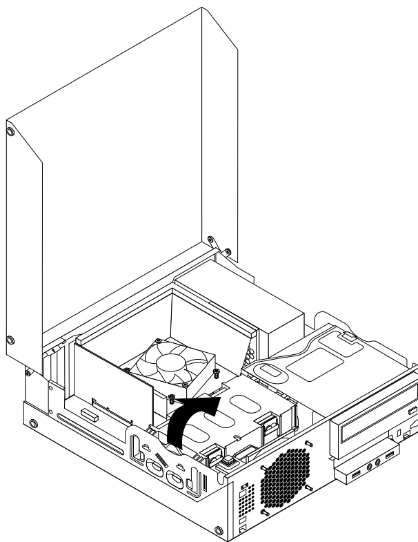
Obrázek 26. Odstranění jednotky pevného disku
