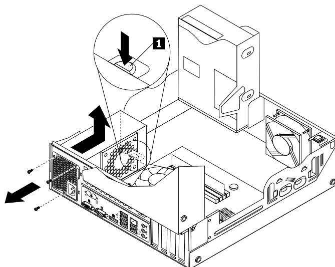
Obrázek 38. Odstranění napájecího zdroje
