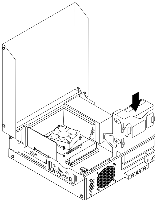
Obrázek 32. Instalace nové optické jednotky
