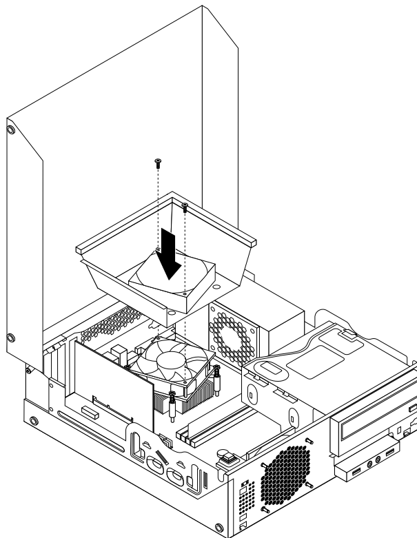
Obrázek 40. Instalace vedení chladiče a větráku
