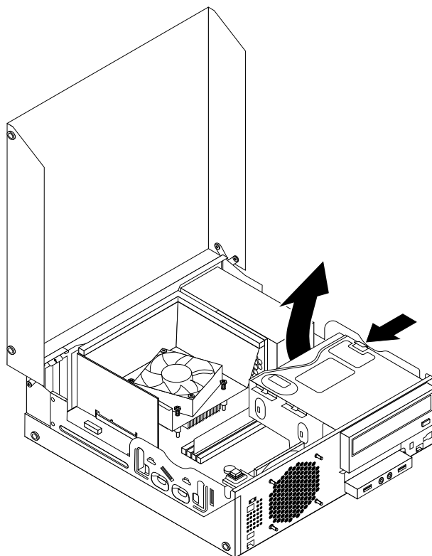
Obrázek 29. Odklopení pozice optické jednotky
