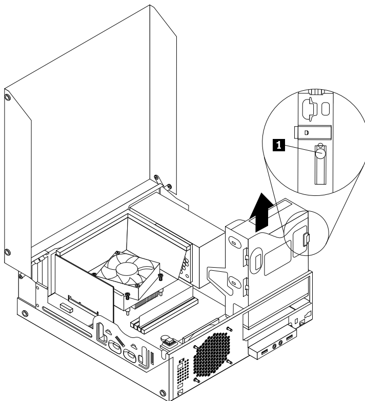
Obrázek 30. Vyjmutí staré optické jednotky
