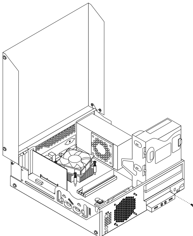
Obrázek 50. Odstranění přední sestavy pro zvuk a USB
