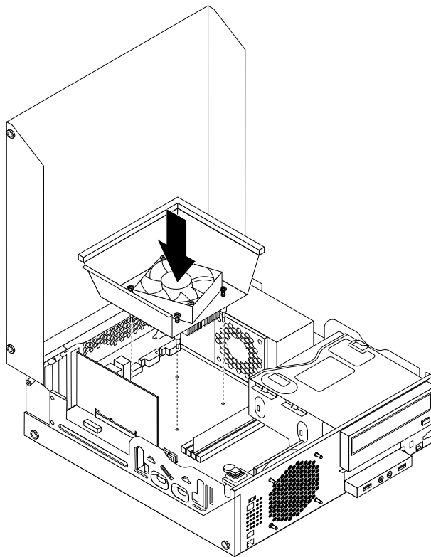
Obrázek 44. Opětovná instalace sestavy chladiče a větráku včetně vedení
