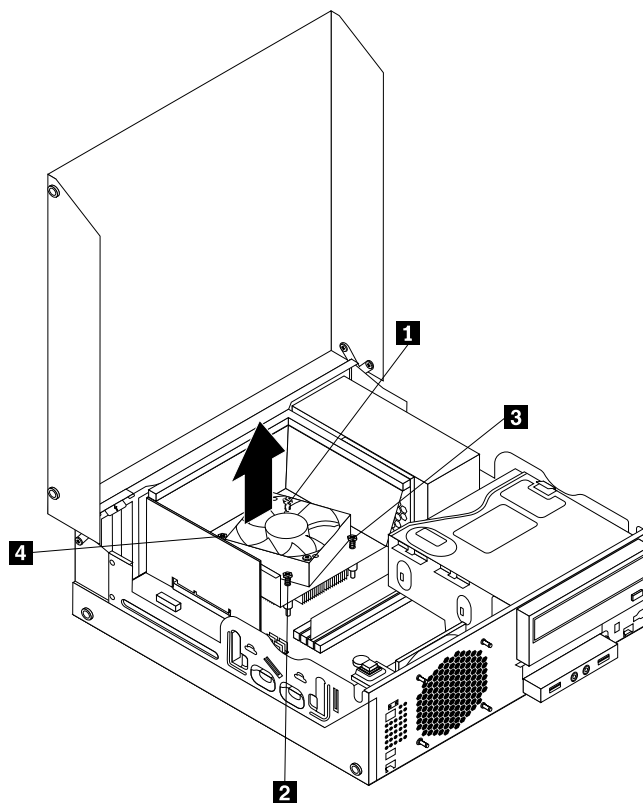
Obrázek 33. Šrouby připevňující sestavu chladiče a větráku
