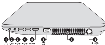
Obrázek 3-6 Pravá strana počítače (X70-A)
