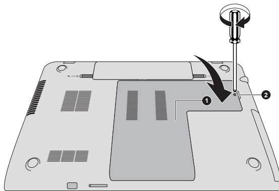
Obrázek 4-15 Usazení krytu paměťového modulu
