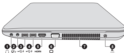
Obrázek 3-5 Pravá strana počítače (P70-A)
