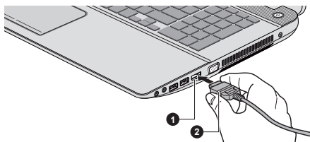
Obrázek 4-20 Připojení výstupního portu HDMI
