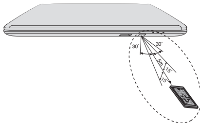
Obrázek 4-3 Provozní rozsah dálkového ovládání
