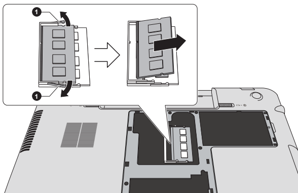
Obrázek 4-16 Vyjmutí paměťového modulu
