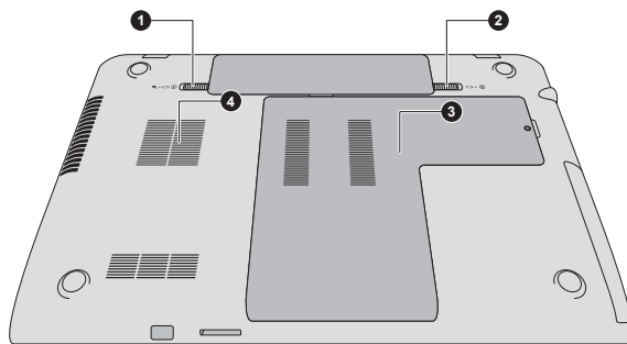
Obrázek 3-8 Spodní strana počítače (P70-A/X70-A)
