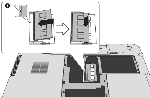
Obrázek 4-14 Usazení paměťového modulu
