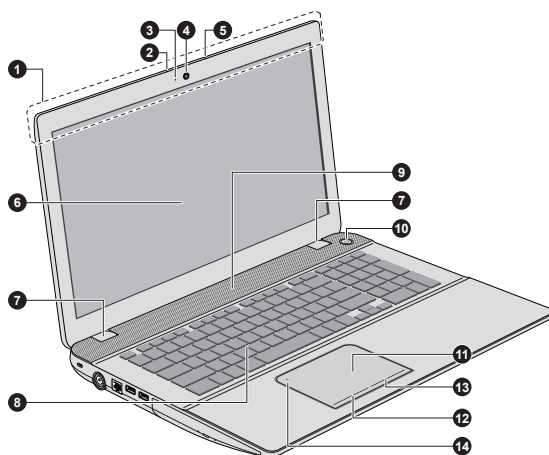
Obrázek 3-10 Přední strana počítače s otevřeným panelem displeje (dotykové modely P70-A/X70-A)
