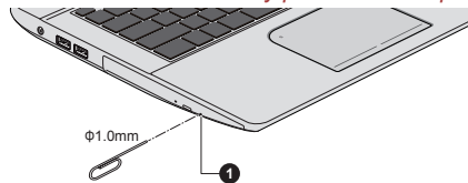
Obrázek 4-4 Ruční otevření zásuvky pomocí otvoru pro vysunutí
