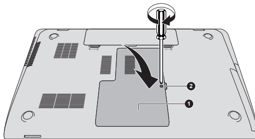
Obrázek 4-10 Usazení krytu paměťového modulu
