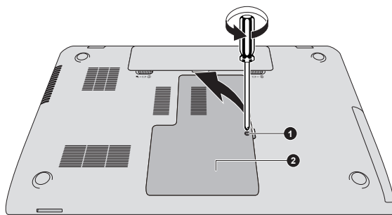
Obrázek 4-8 Sejmutí krytu paměťového modulu
