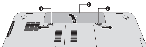
Obrázek 4-5 Uvolnění baterie - 1
