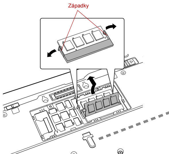
Obrázek 3-10 Vyjmutí paměťového modulu
