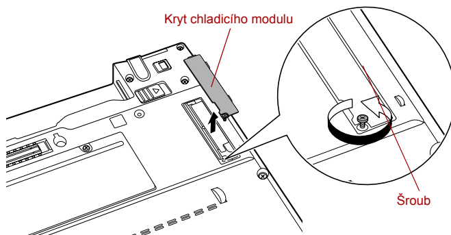
Obrázek G-1 Vyjmutí krytu chladicího modulu
