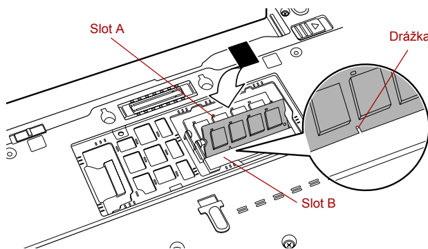
Obrázek 3-8 Usazení paměťového modulu
