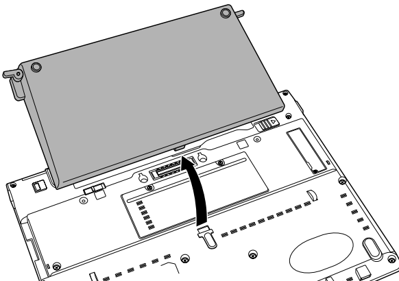
Obrázek 6-6 Vyjmutí tenké přídatné baterie
