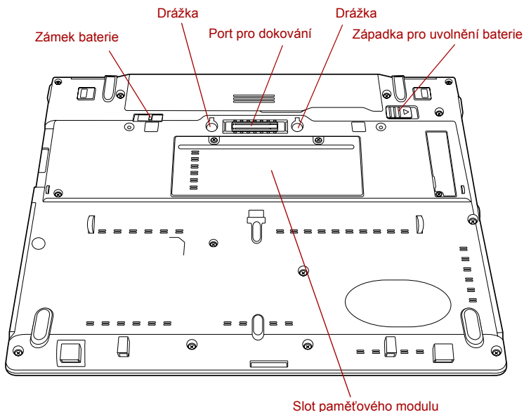
Obrázek 2-5 Spodní strana počítače
