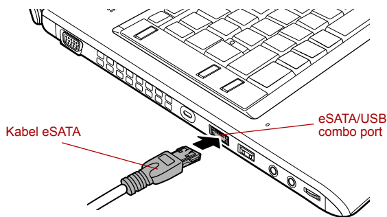
Obrázek 3-14 Připojení kabelu eSATA do combo portu eSATA/USB
