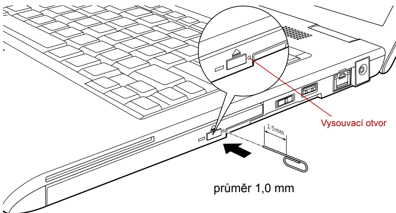
Obrázek 4-8 Ruční otevření zásuvky pomocí otvoru pro vysunutí
