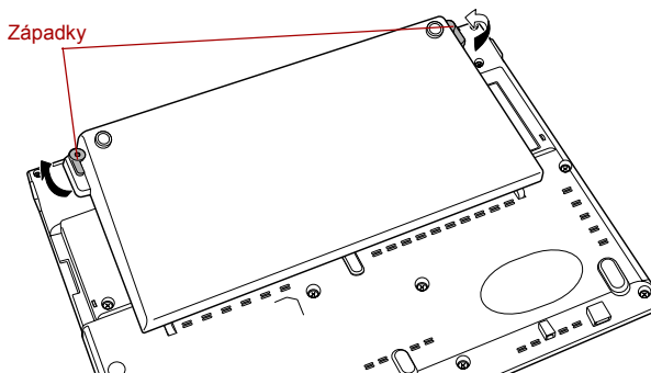
Obrázek 6-5 Uvolnění západek
