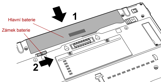
Obrázek 6-2 Zabezpečení baterie
