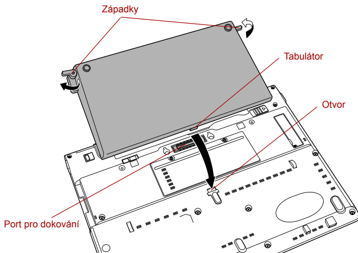
Obrázek 6-3 Usazení tenké přídatné baterie
