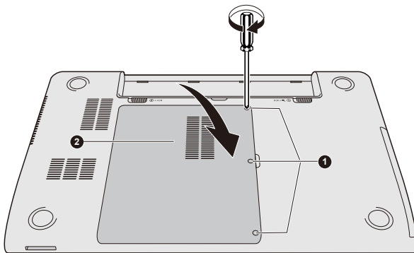
Obrázek 3-12 Usazení krytu paměťového modulu
