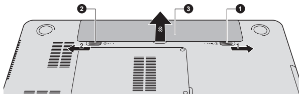
Obrázek 5-1 Uvolnění baterie - 1
