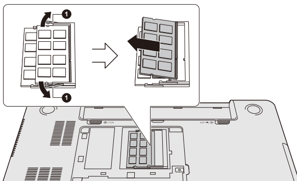
Obrázek 3-13 Vyjmutí paměťového modulu
