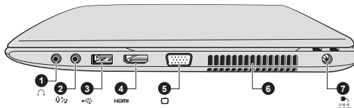
Obrázek 2-3 Pravá strana počítače
