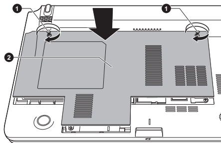
Obrázek 3-13 Usazení krytu paměťového modulu
