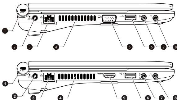
Obrázek 2-2 Levá strana počítače
