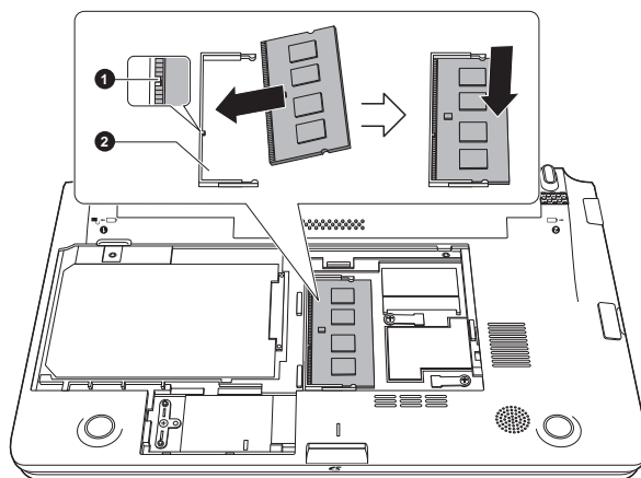
Obrázek 3-12 Usazení paměťového modulu
