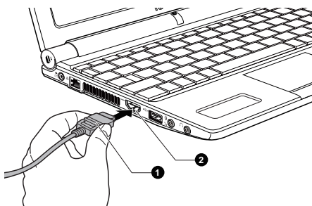
Obrázek 3-15 Připojení výstupního portu HDMI
