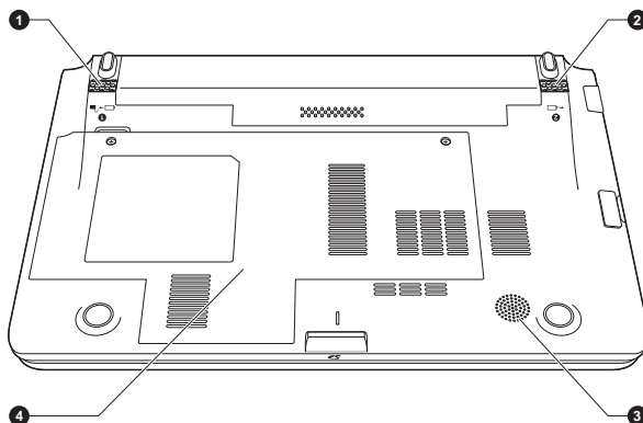
Obrázek 2-5 Spodní strana počítače
