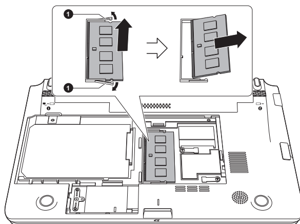
Obrázek 3-10 Vyjmutí paměťového modulu
