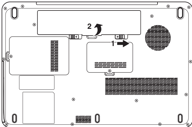
Obrázek 6-2 Uvolnění baterie (2)
