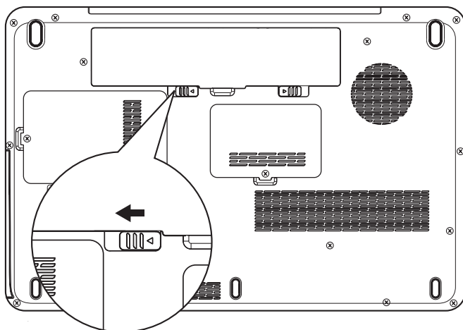
Obrázek 6-1 Uvolnění baterie (1)
