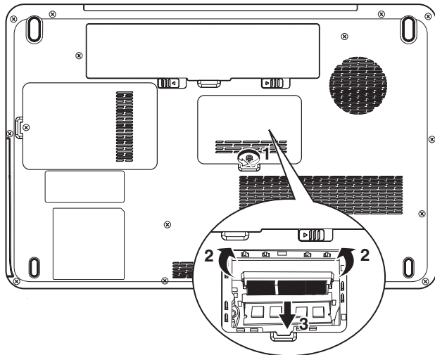
Obrázek 8-2 Sejmутí krytu paměťového modulu
